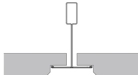
Reveal Edge
